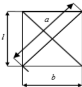
Рисунок 5 – Схема крестовой решетки с распорками
