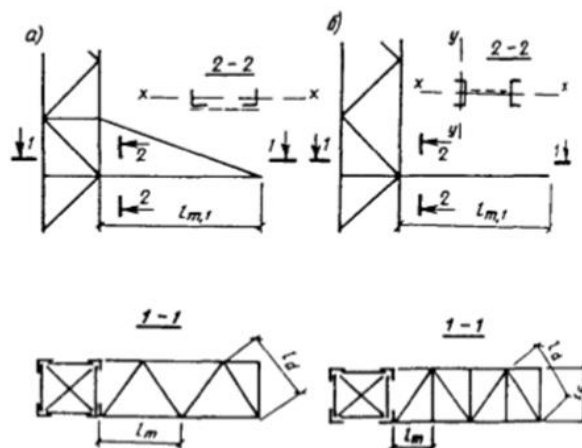
24-сүрөт – Траверс үлгүлөрү
