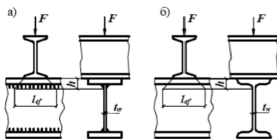
б-сүрөт – Устундуга жүкөмдү бөлүштүрүүнүн узундугун аныктоо үчүн схемалар а – шитерилген б – прокат
